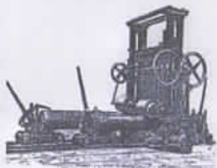
"Den industrialiserede Husmands" tømmer-sæve-maskine.
